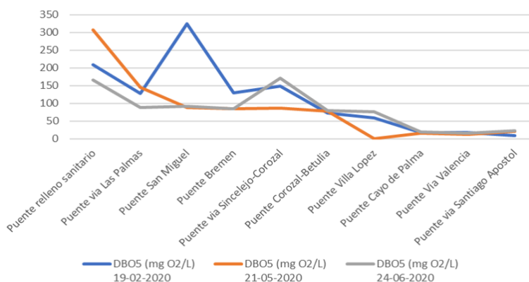
Resultados de la concentración de DBO en la microcuenca del arroyo Grande de Corozal - LCAMorrosquillo
