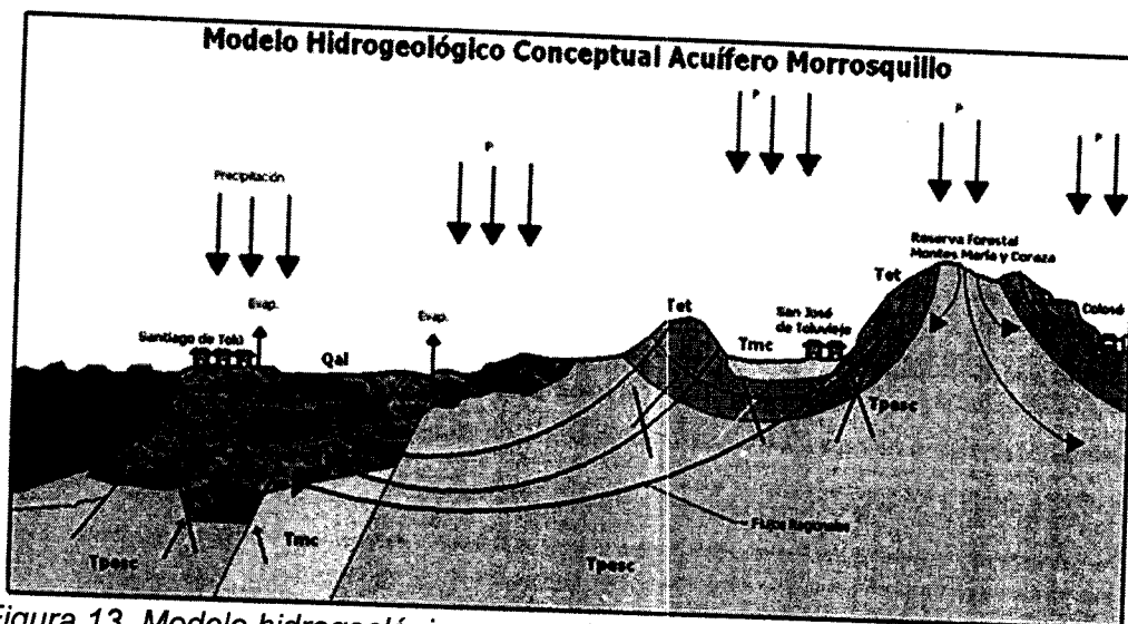
Figura 13. Modelo hidrogeológico conceptual del acuífero Morrosquillo. Fuente: CARSUCRE, (2011).
